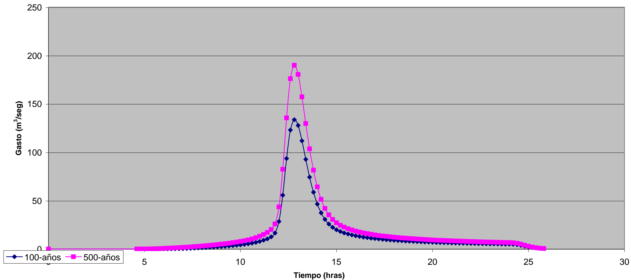
GRÁFICA 3.15 Hidrograma Qda. Enlozada 100- y 500-años
