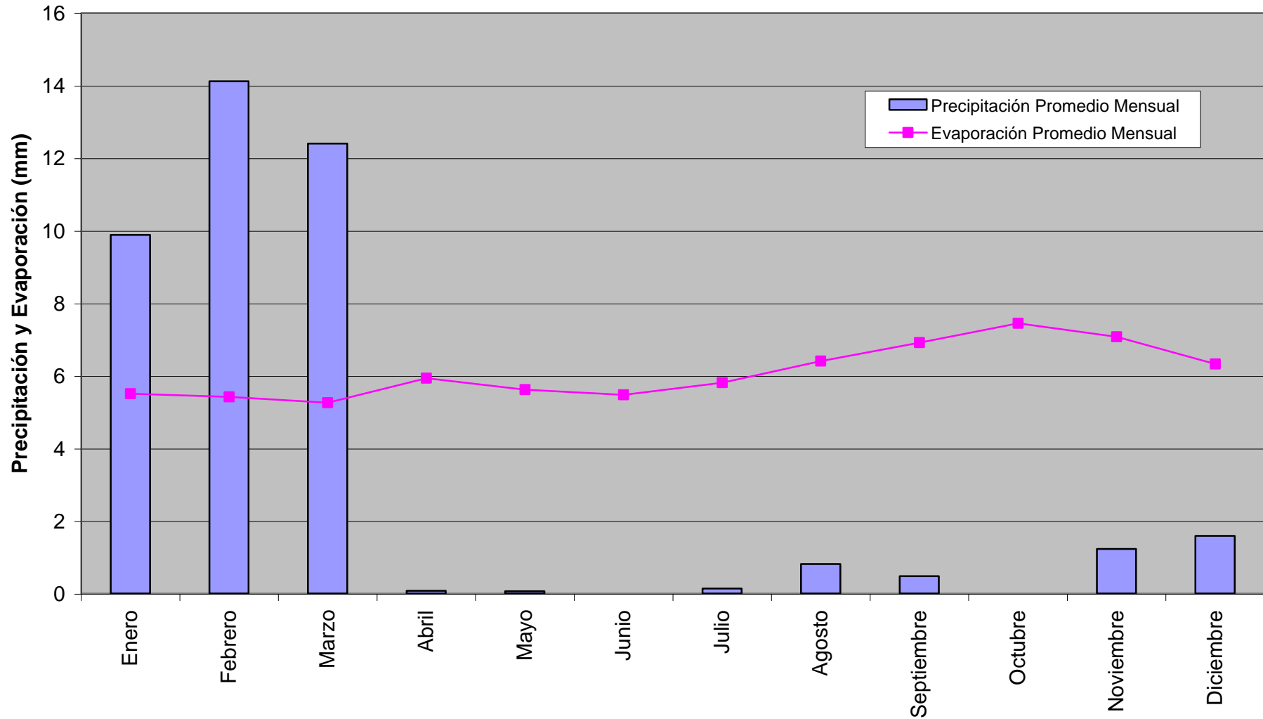
GRÁFICA 3.1 Relación entre Precipitación Promedio Mensual y Evaporación Estación Meteorológica Cerro Verde Sur (1995 - 2002)
