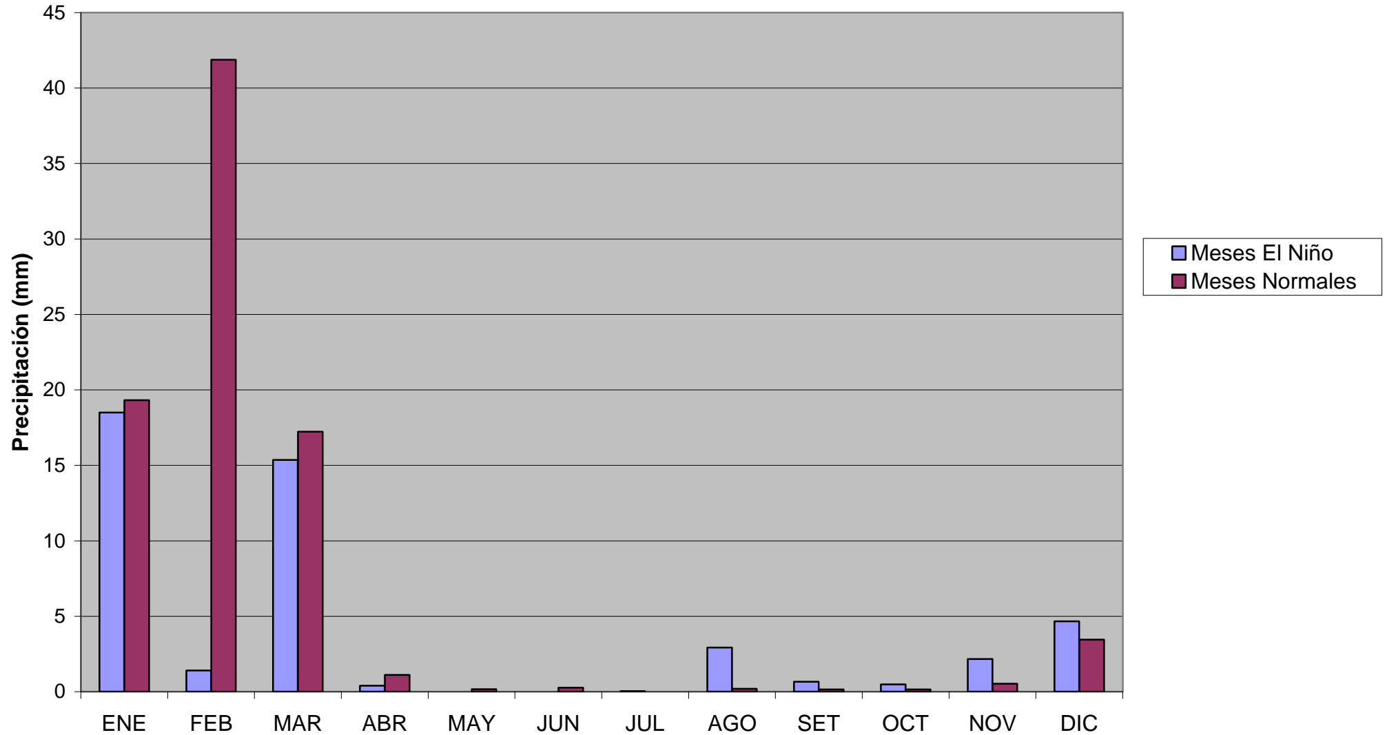
GRÁFICA 3.2 Comparación Promedio Mensual de "Meses Niño" y "Meses Normales" - Anual (1980 - 2001) Estación Meteorológica La Pampilla
