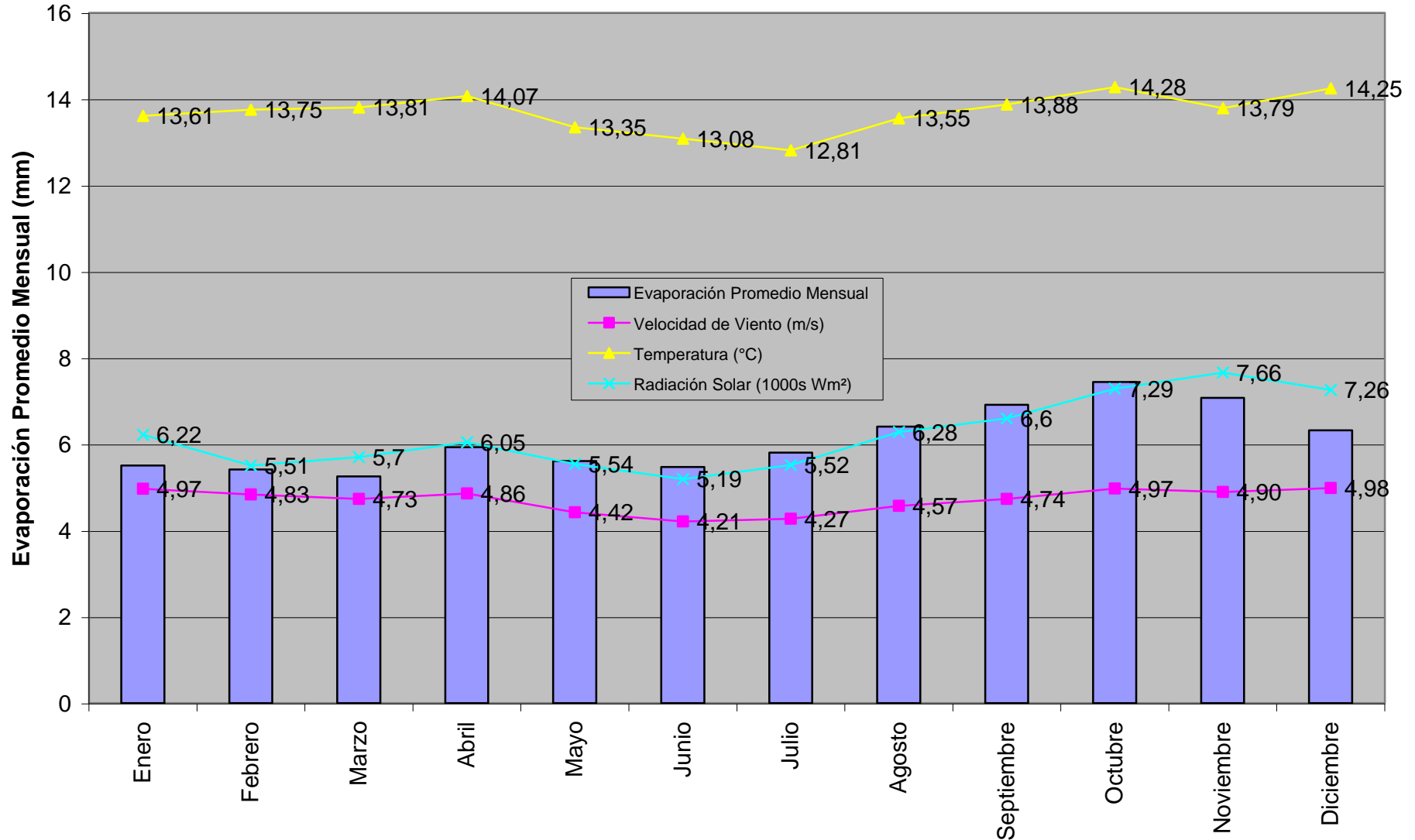
GRÁFICA 3.8 Relación entre Evaporación Promedio Mensual, Velocidad del Viento, Temperatura Promedio Mensual y Radiación Solar
