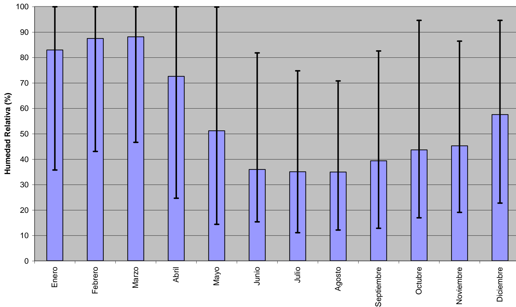
GRÁFICA 3.7 Distribución Anual de la Humedad Relativa (1995 - 2002) Estación Meteorológica Cerro Verde Sur
