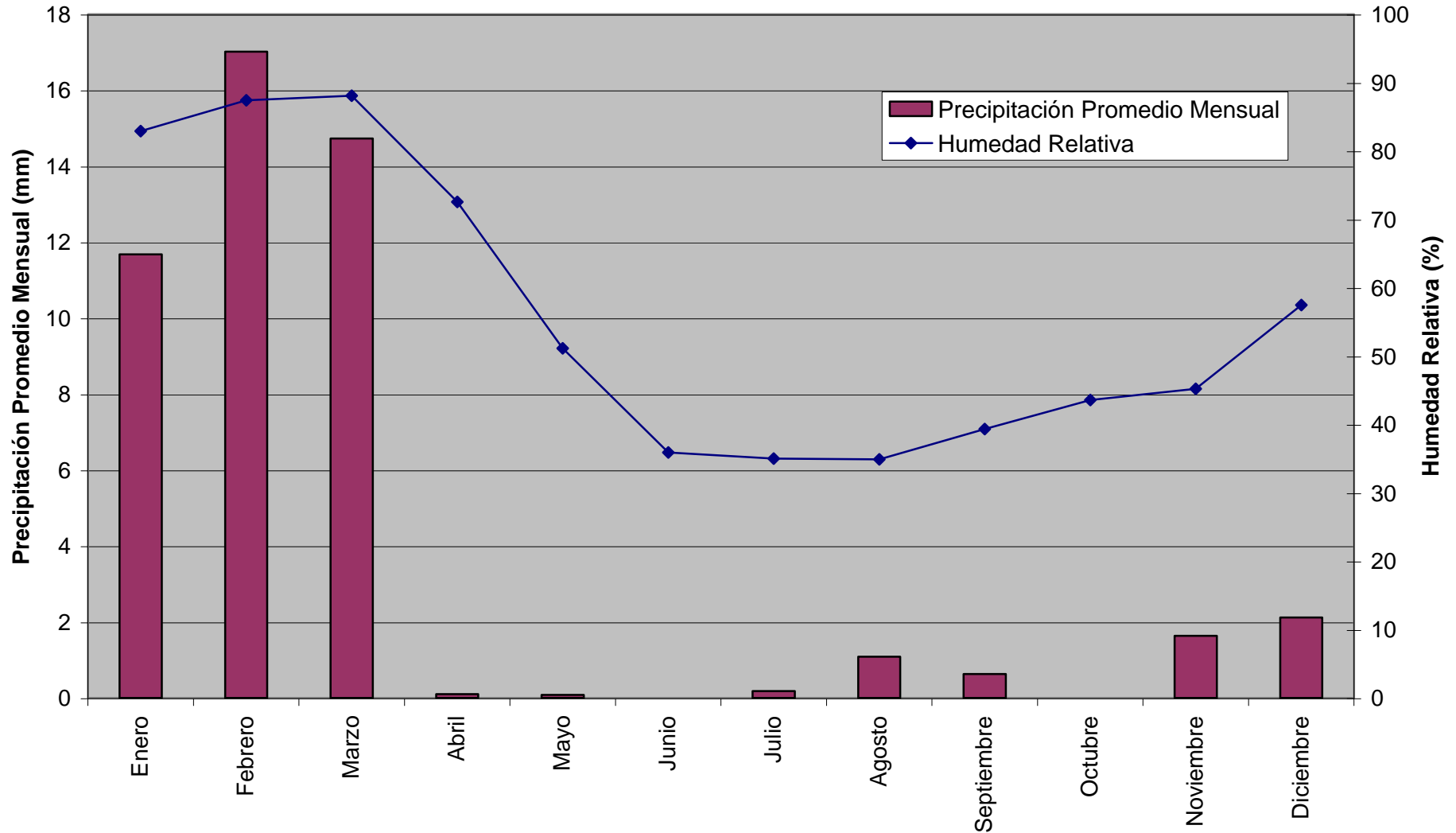
GRÁFICA 3.6 Relación entre Precipitación y Humedad Relativa (1995 - 2002) Estación Meteorológica Cerro Verde Sur
