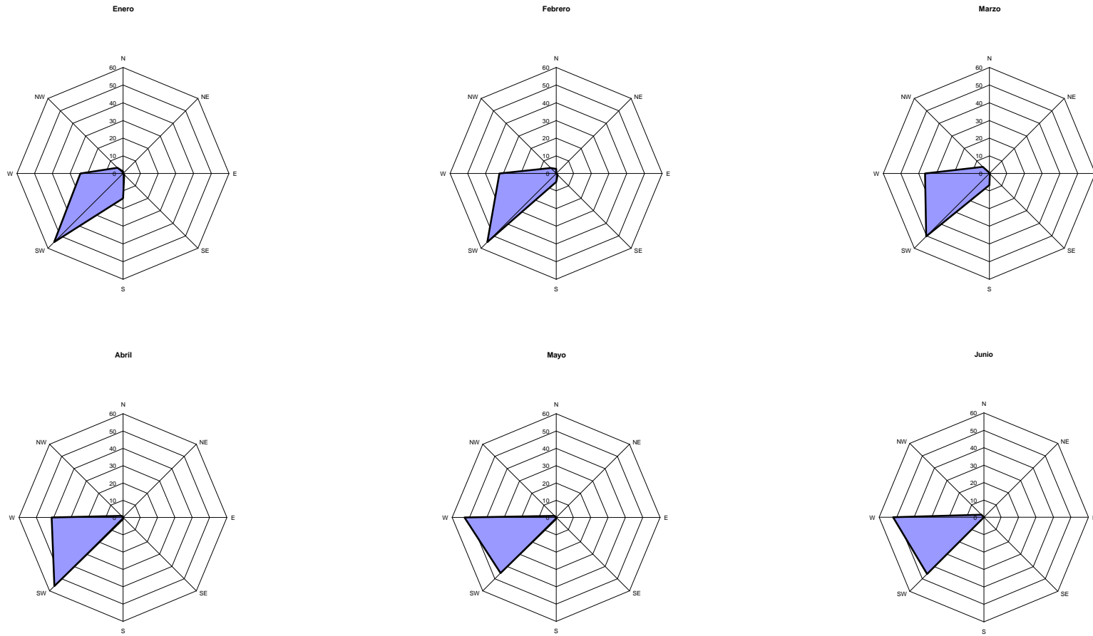
GRÁFICA 3.11 Dirección de Viento - Meses de Enero a Junio (1995 -2002) – Estación Meteorológica Cerro Verde Sur
