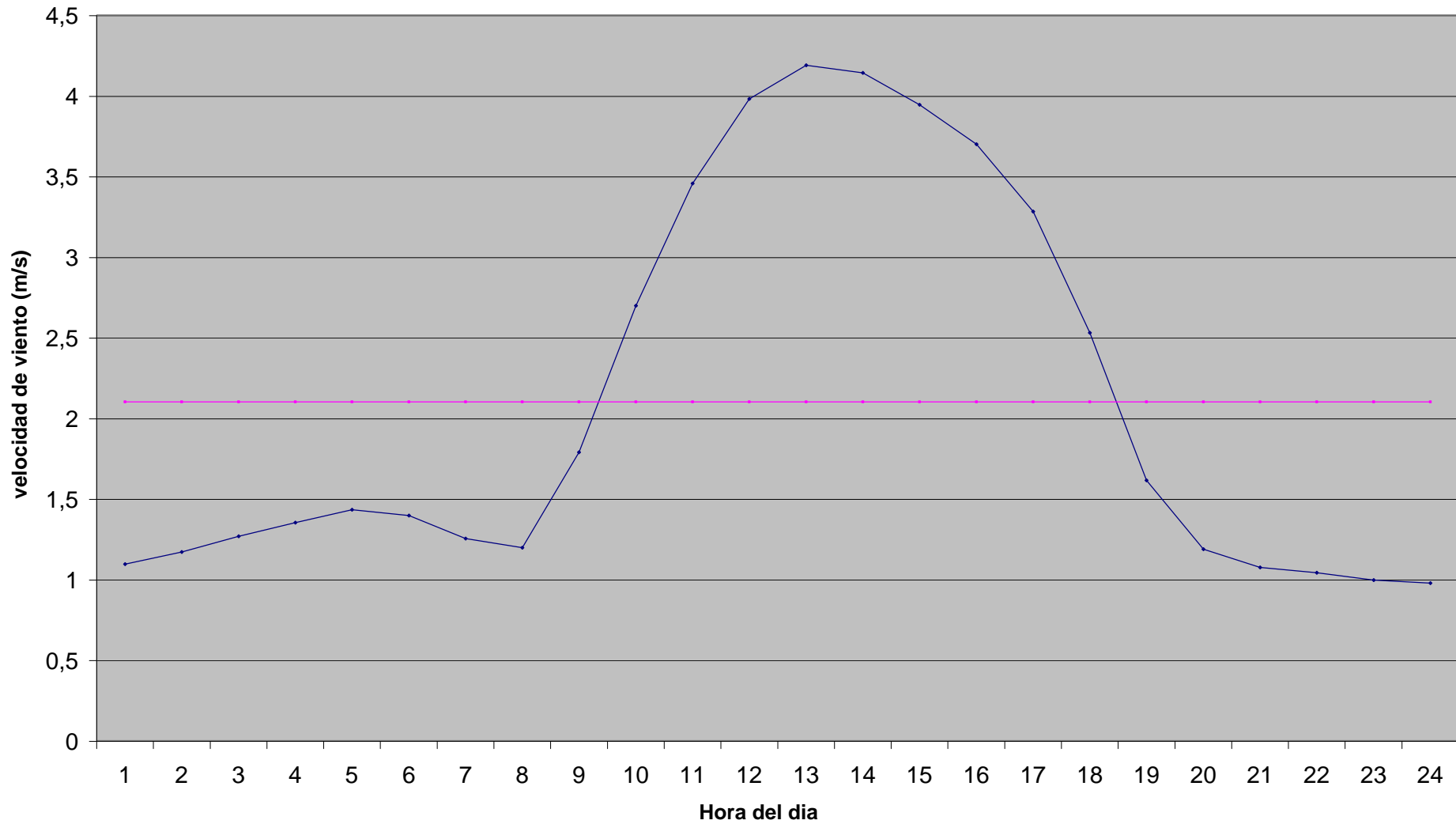
Comportamiento de la velocidad del viento a lo largo del día
