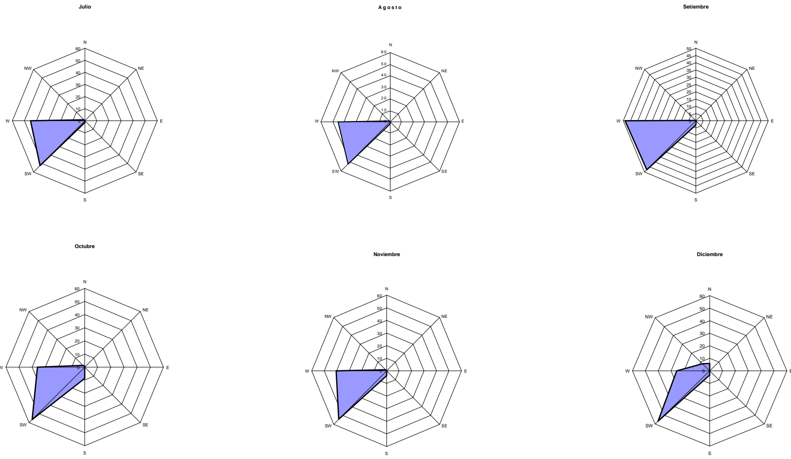
GRÁFICA 3.12 Dirección de Viento - Meses de Julio a Diciembre (1995 -2002) – Estación Meteorológica Cerro Verde Sur
