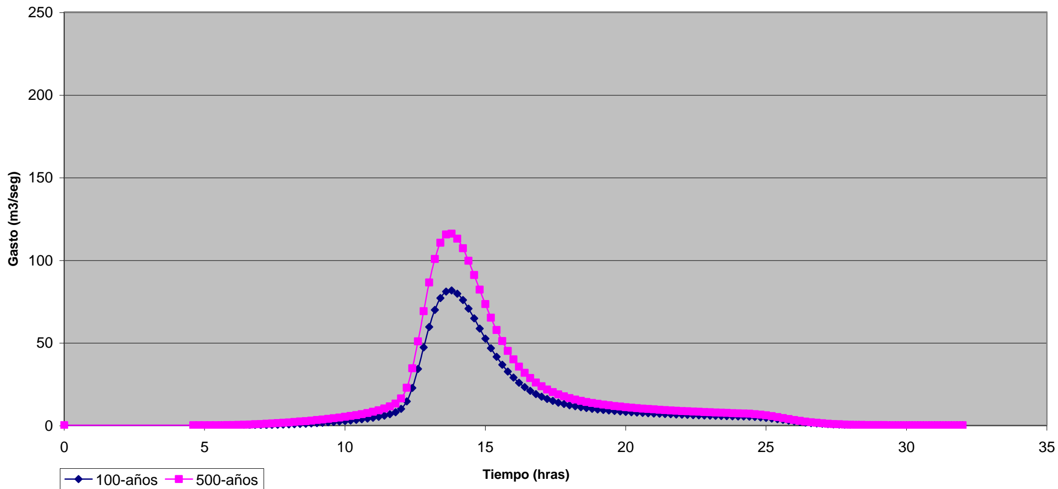
GRÁFICA 5.3 Hidrograma de Qda. Enlozada 100- y 500-años (en cierre)
