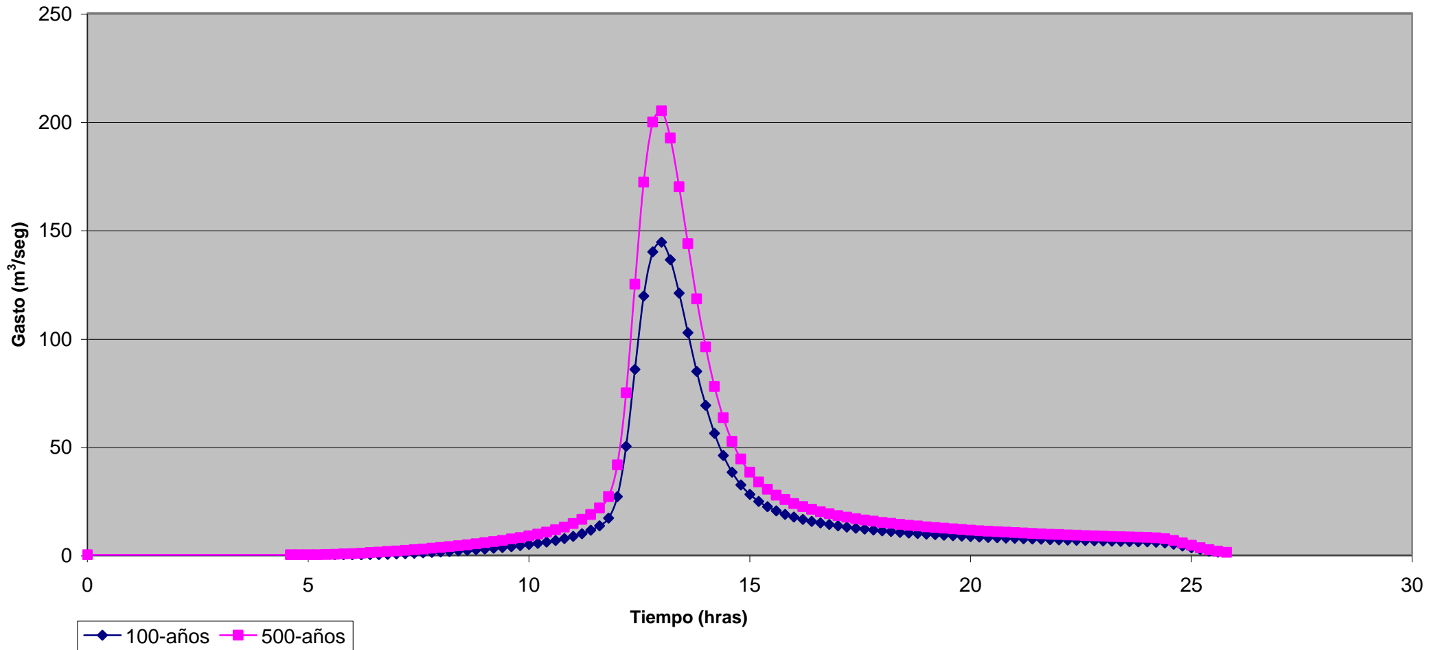
GRÁFICA 5.4 Hidrograma Qda. Tinajones 100- y 500-años (en cierre)
