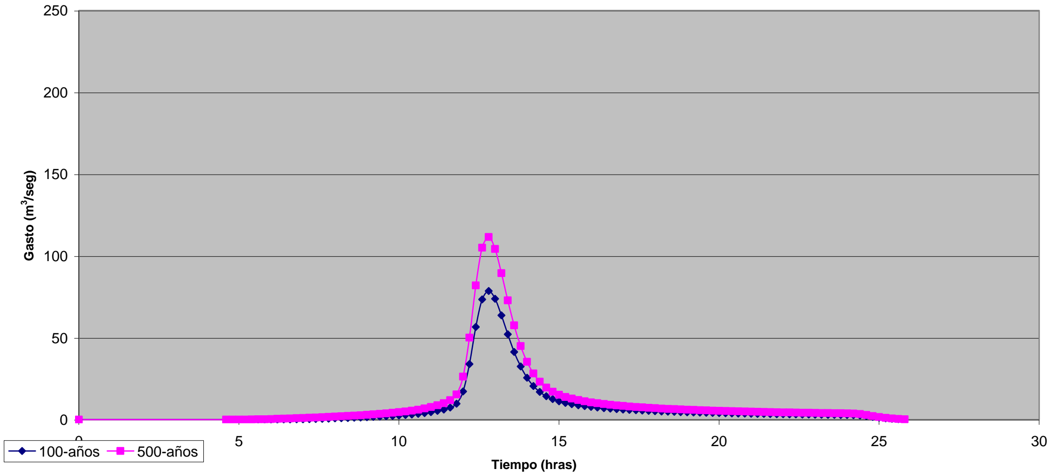
GRÁFICA 5.2 Hidrograma de Qda. Enlozada 100- y 500-años (en cierre)
