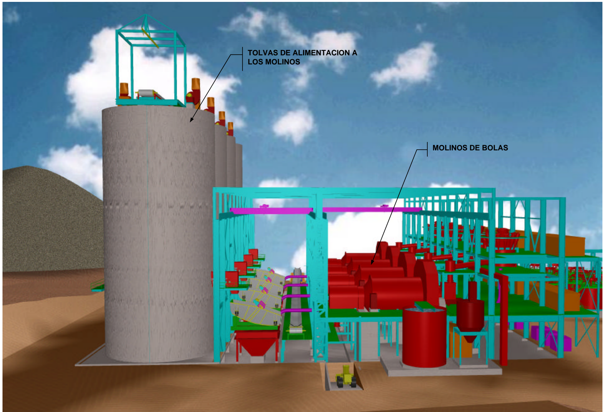
Figura 4.7 Arreglo General del Circuito de Molienda con Molinos de Bolas
