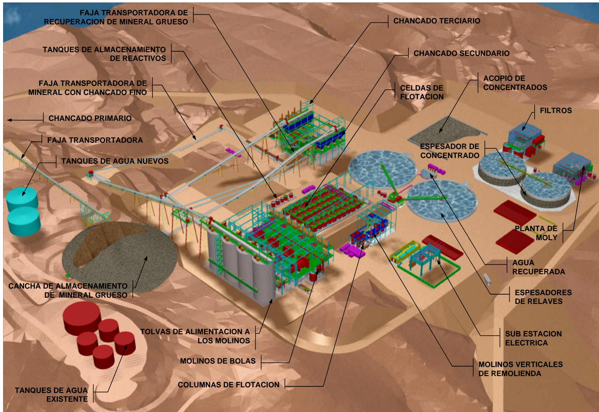
Figura 4.5 Arreglo Tridimensional del Sistema de Acopio de Mineral Grueso y Planta Concentradora
