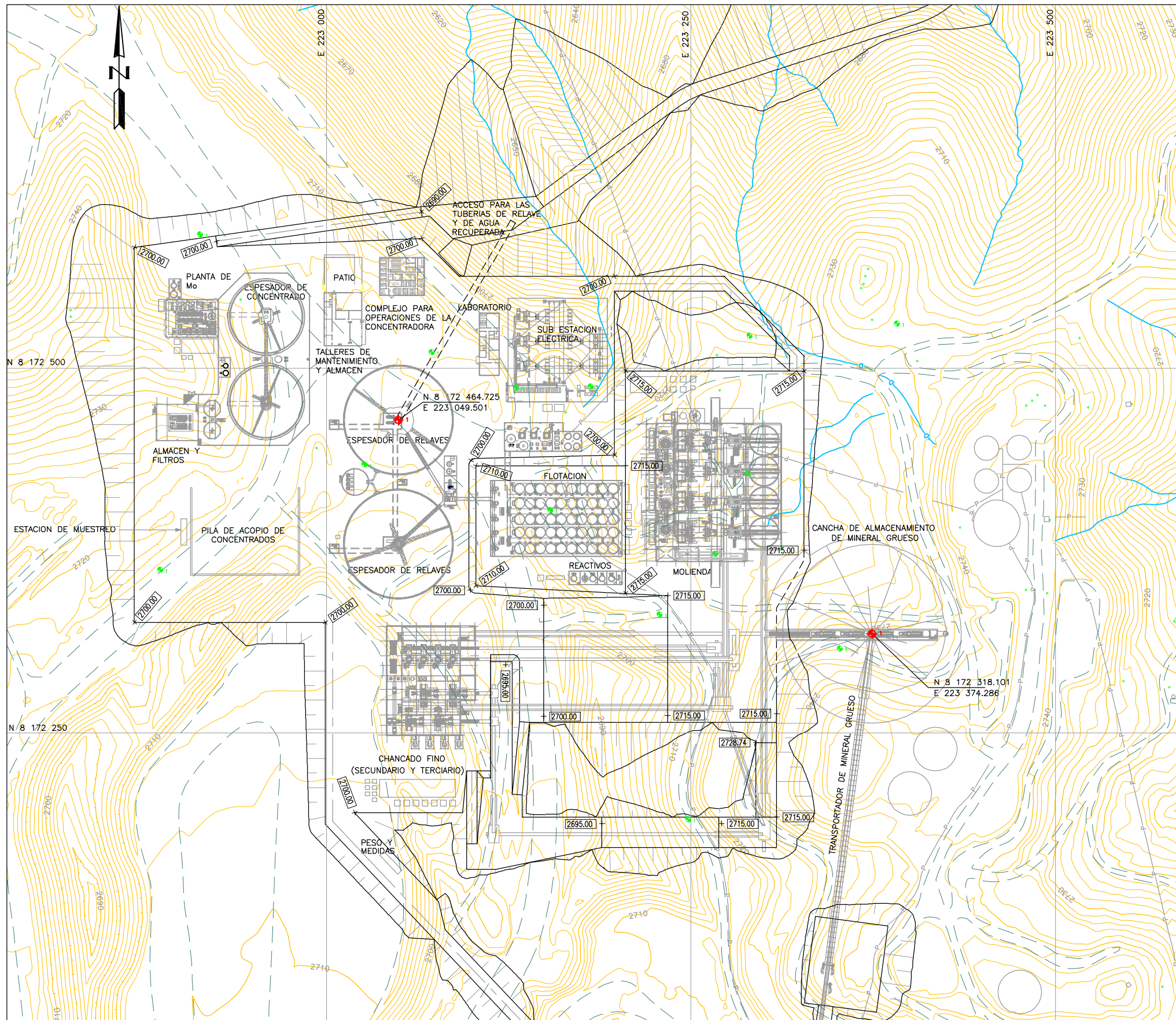
PLANTA 30 0 30 60 METROS SCALE = 1:1500
